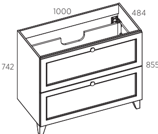
VALAMUKAPP 100
