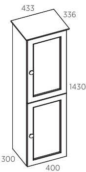
KÜLJEKAPP
