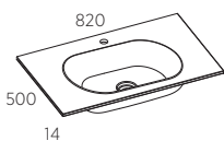
VALAMUKAPP 80
