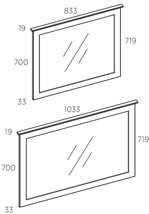
MDF-RAAMIGA PEEGEL 80/100
