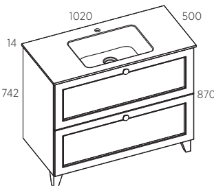
VALAMUKAPP+LETTVALAMU 100
