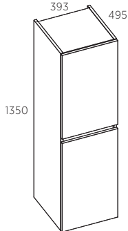
VALGUSTUSEGA KAPP
