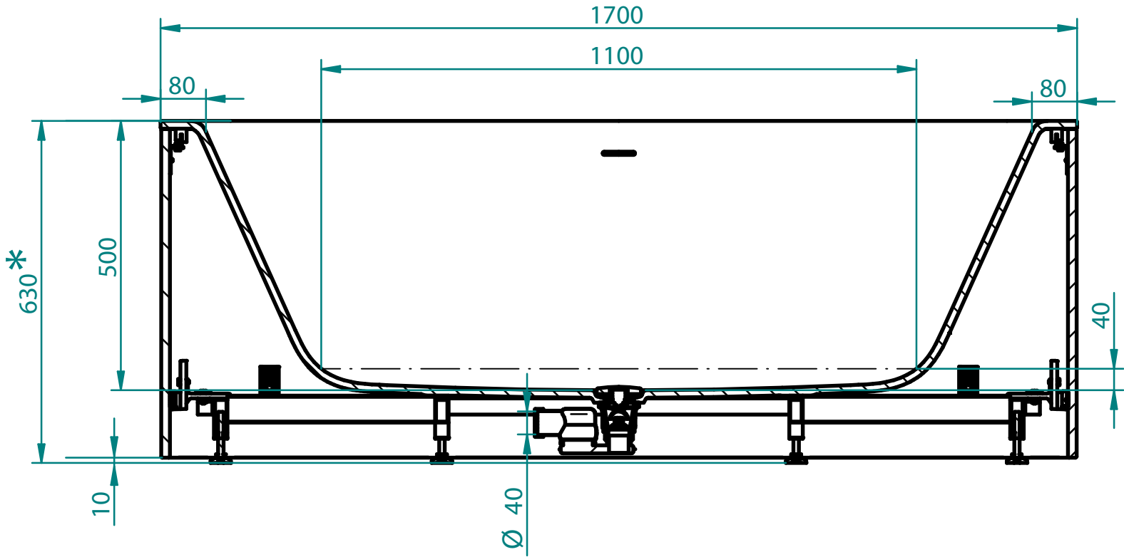
SECTION A-A
