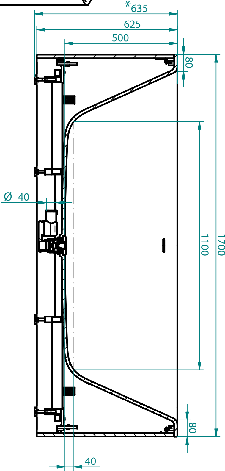
SECTION A-A
